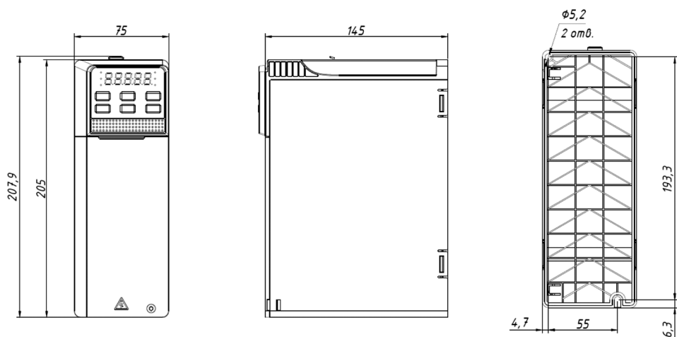
Рис. 3.6-2. Чертеж преобразователя частоты типоразмера C2
