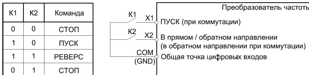
Рисунок 8.8-2 – Двухпроводная схема управления 2
