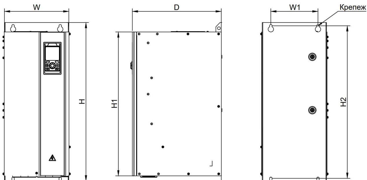
Рисунок 3.6-3 Чертеж преобразователя частоты типоразмеров M6-M11
