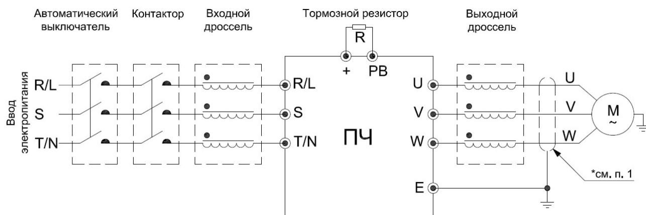
Рисунок 4.3-1 – Схема подключения преобразователя частоты
