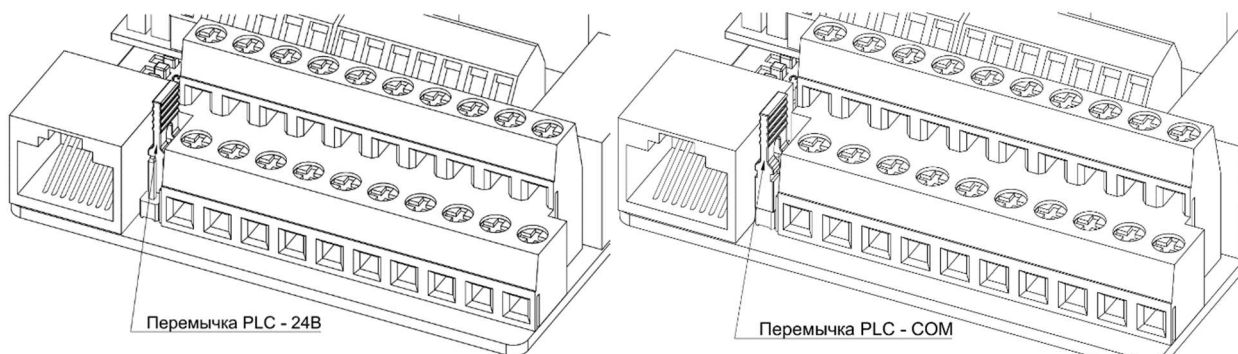
Рисунок 4.6-1 - Способ подключения логики PNP и NPN
