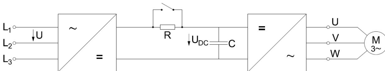
Рисунок 1.5-1 – Схема силовой части преобразователя частоты с промежуточным звеном постоянного тока
