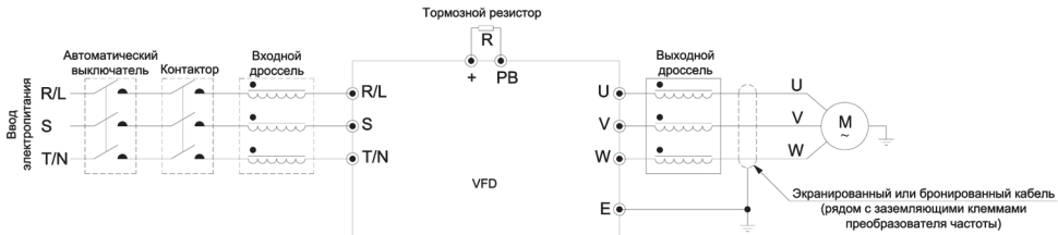
Рисунок 3.1-1. Схема подключения преобразователя частоты
