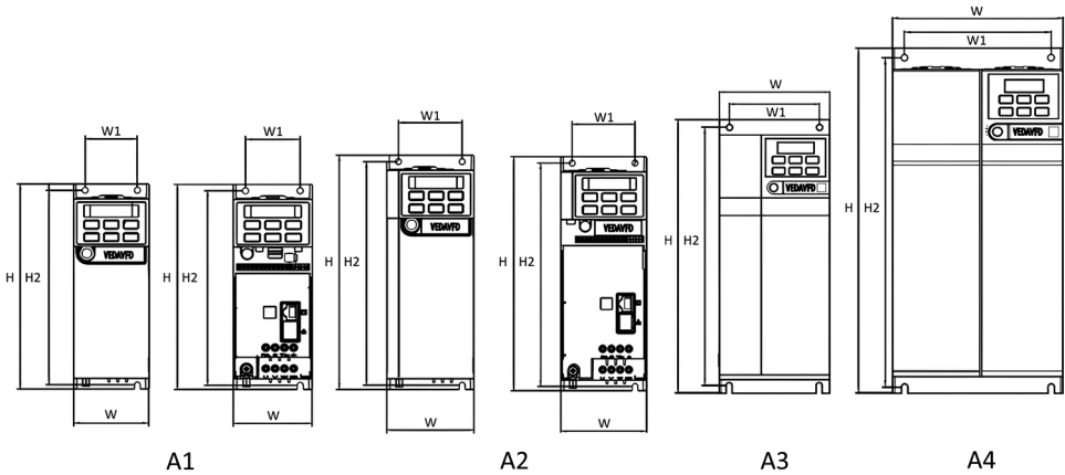
Рисунок 2.1-1. Типоразмеры преобразователей частоты
