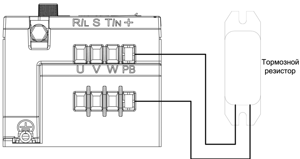
Рисунок 3.3-1. Подключение тормозного резистора для преобразователей частоты VF-51
