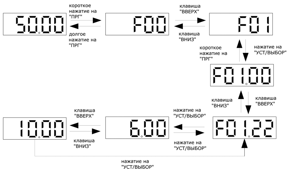
Рисунок 4.2-1. Базовые операции на панели управления
