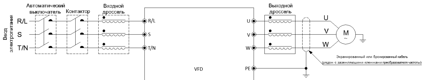
Рисунок 3.4-1 Схема подключения преобразователя частоты
