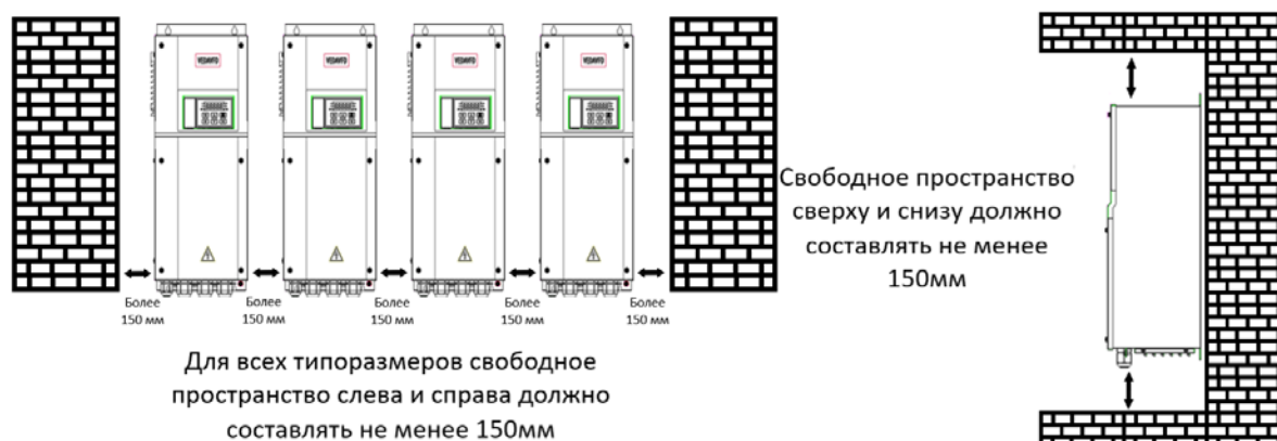
Рисунок 2.5-1 Рекомендуемые монтажные расстояния
