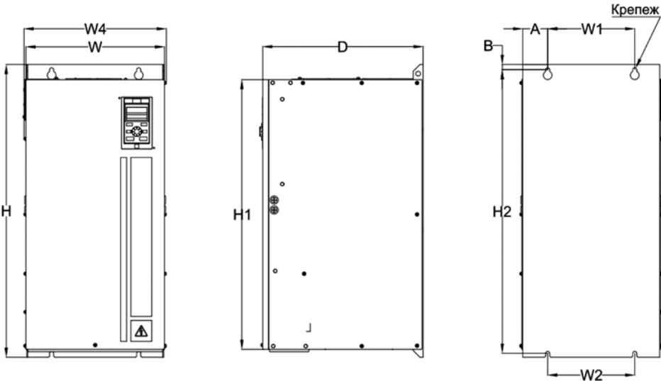
Рисунок 3.6-8 – Чертеж преобразователя частоты типоразмера B8
