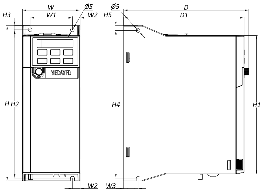
Рисунок 3.6-3 – Чертеж преобразователя частоты типоразмера A2 с защитной крышкой
