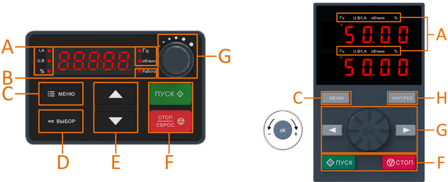
Рисунок 5.3-1 – Панель управления преобразователя частоты
