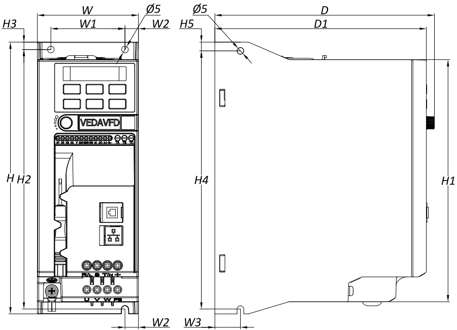
Рисунок 3.6-4 – Чертеж преобразователя частоты типоразмера A2 без защитной крышки
