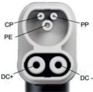
Схема 8.2 Схема положения контактов вилки разъема постоянного тока транспортного средства на выходе
