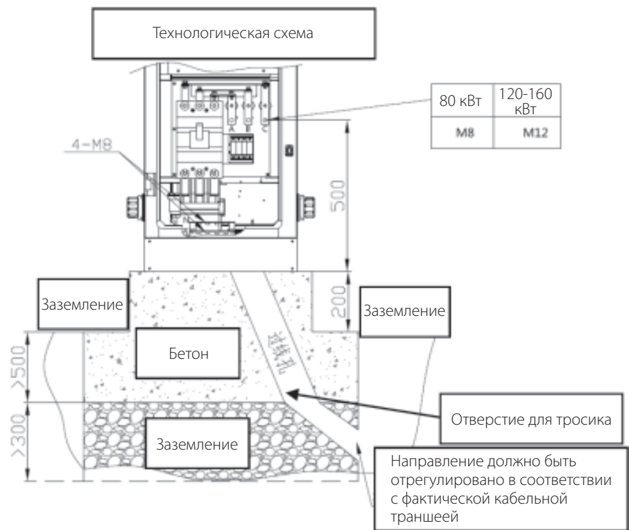
Рисунок 7.2.1 Строительный чертеж
