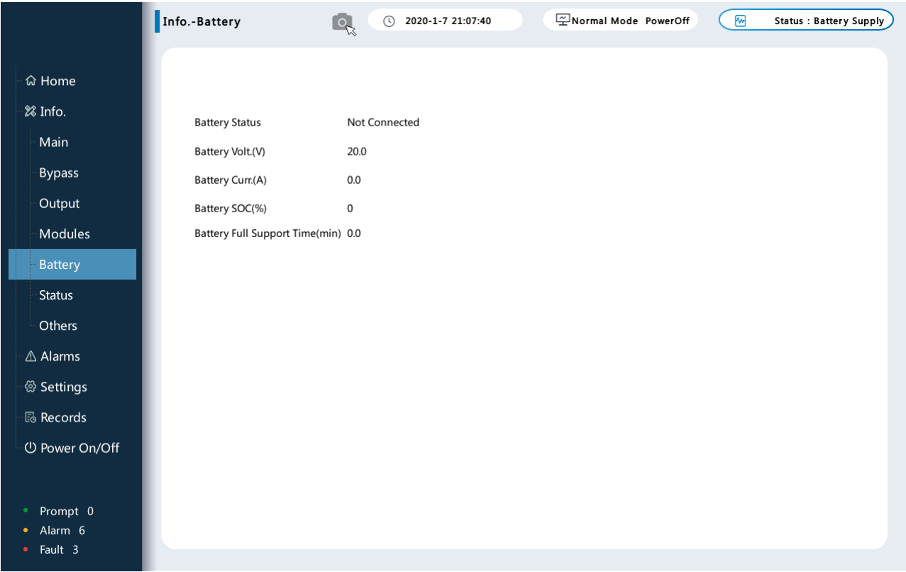
Рисунок 5-7 Экран аккумулятора
