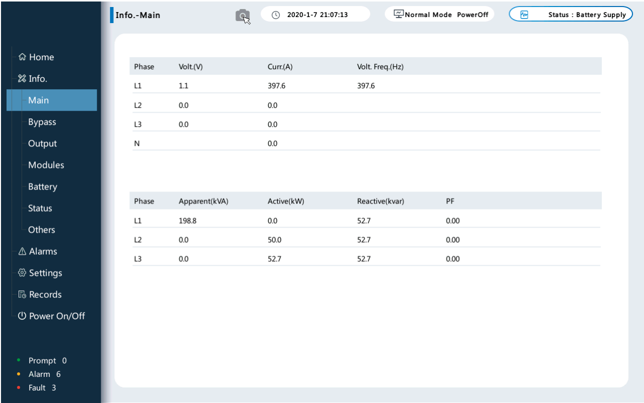
Рисунок 5-2 Главный экран
