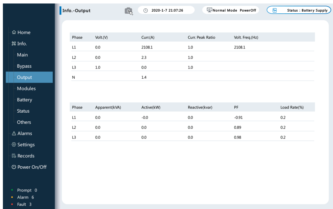
Рисунок 5-4 Экран вывода
