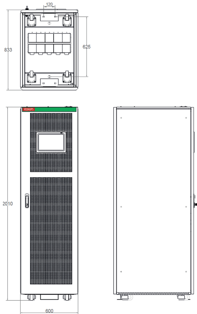
Рисунок 4-1 Таблица физических размеров ИБП
