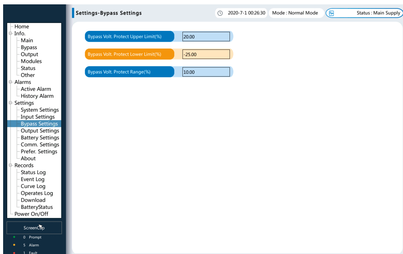
Рисунок 5-15 Настройки байпаса
