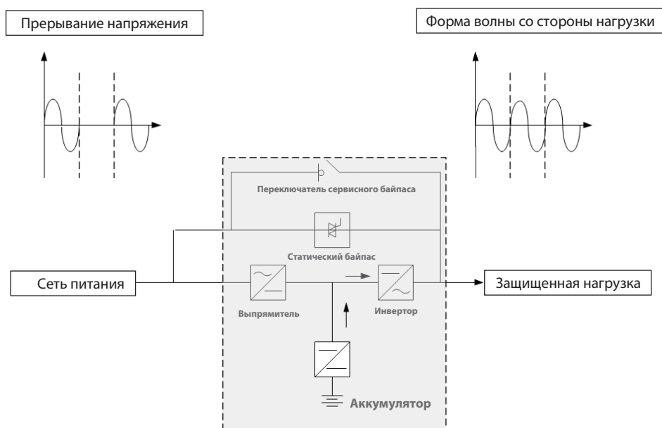
Рисунок 2-2 Схема управления при прерывании напряжения
