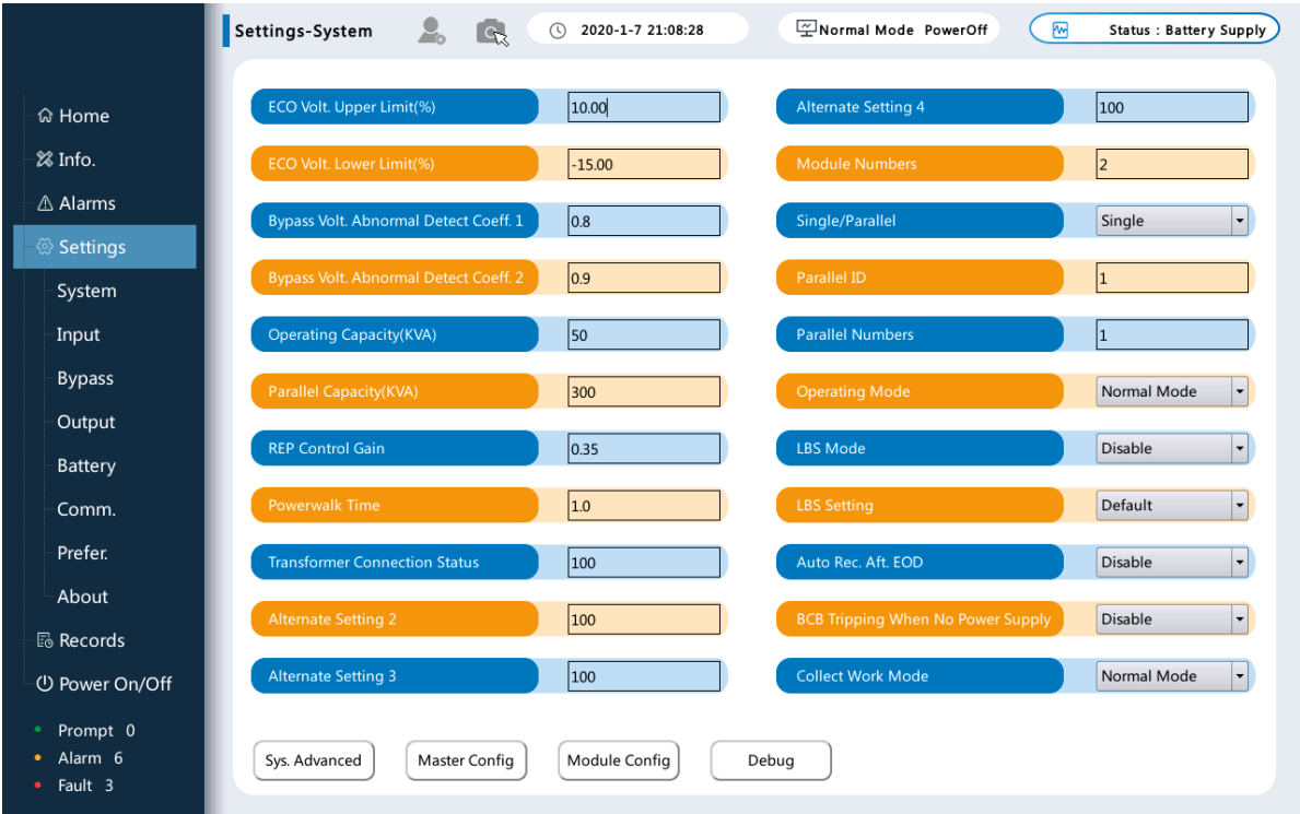
Рисунок 5-13 Настройки системы
