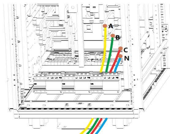
Рисунок 4-6 Выходное подключение
