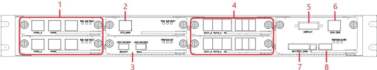
Рисунок 3-10 Внешний вид главного модуля управления
