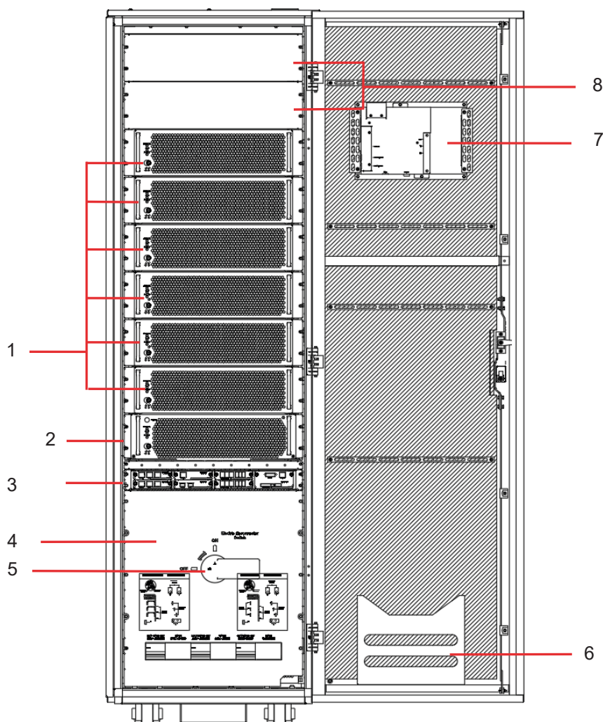
Рисунок 3-2 VEDAUPS 300, вид спереди
